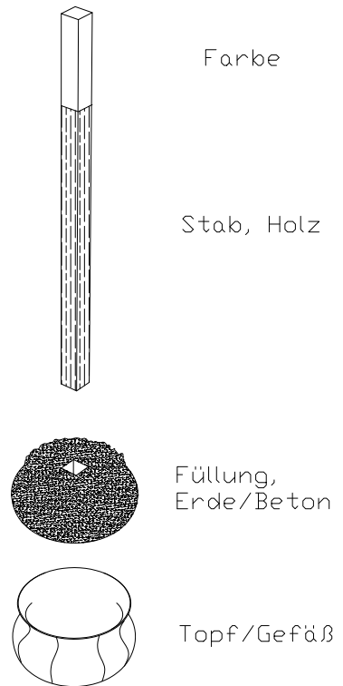
Explosionsgrafik Holzstele in Topf
