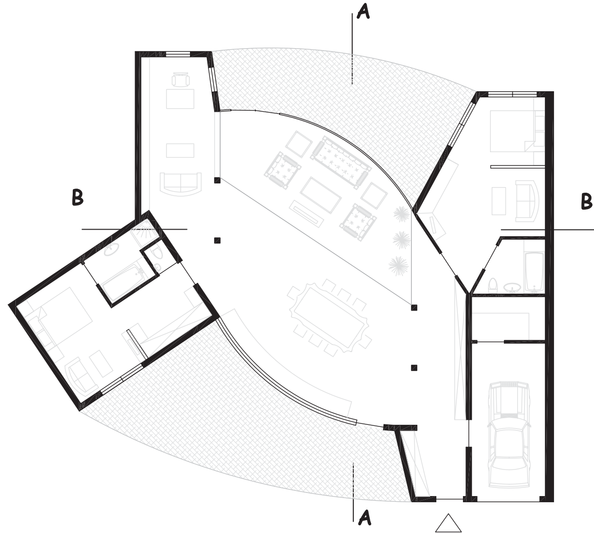
Grundriss neu
